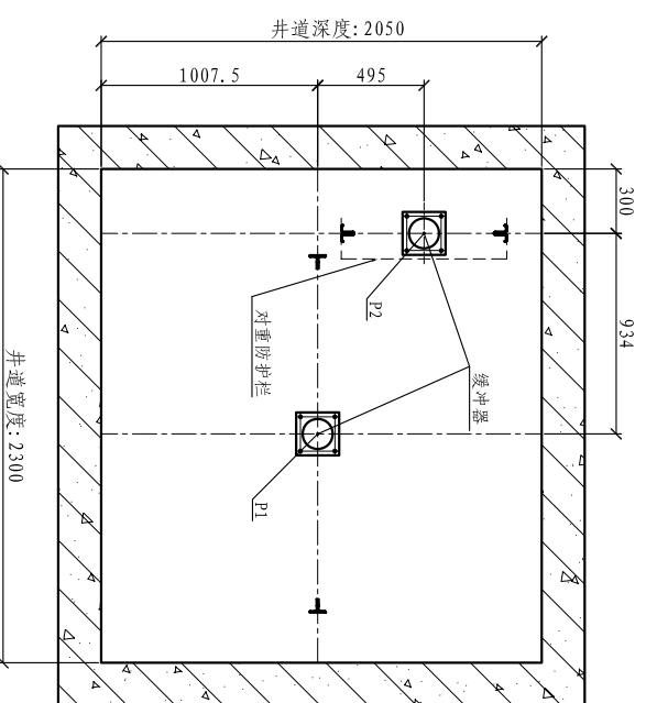
底坑平面布置图
